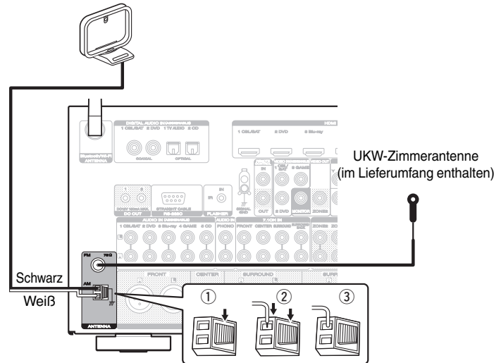
MW-Rahmenantenne (im Lieferumfang enthalten)
